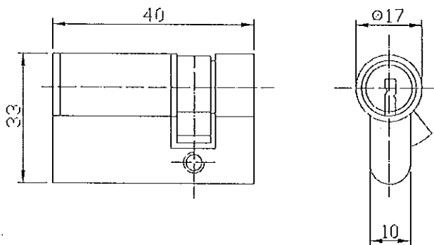
Фигура 1 - Патрон халф цилиндър със секрет
